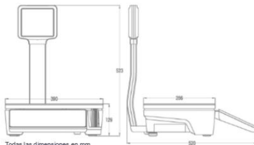
Todas las dimensiones en mm
